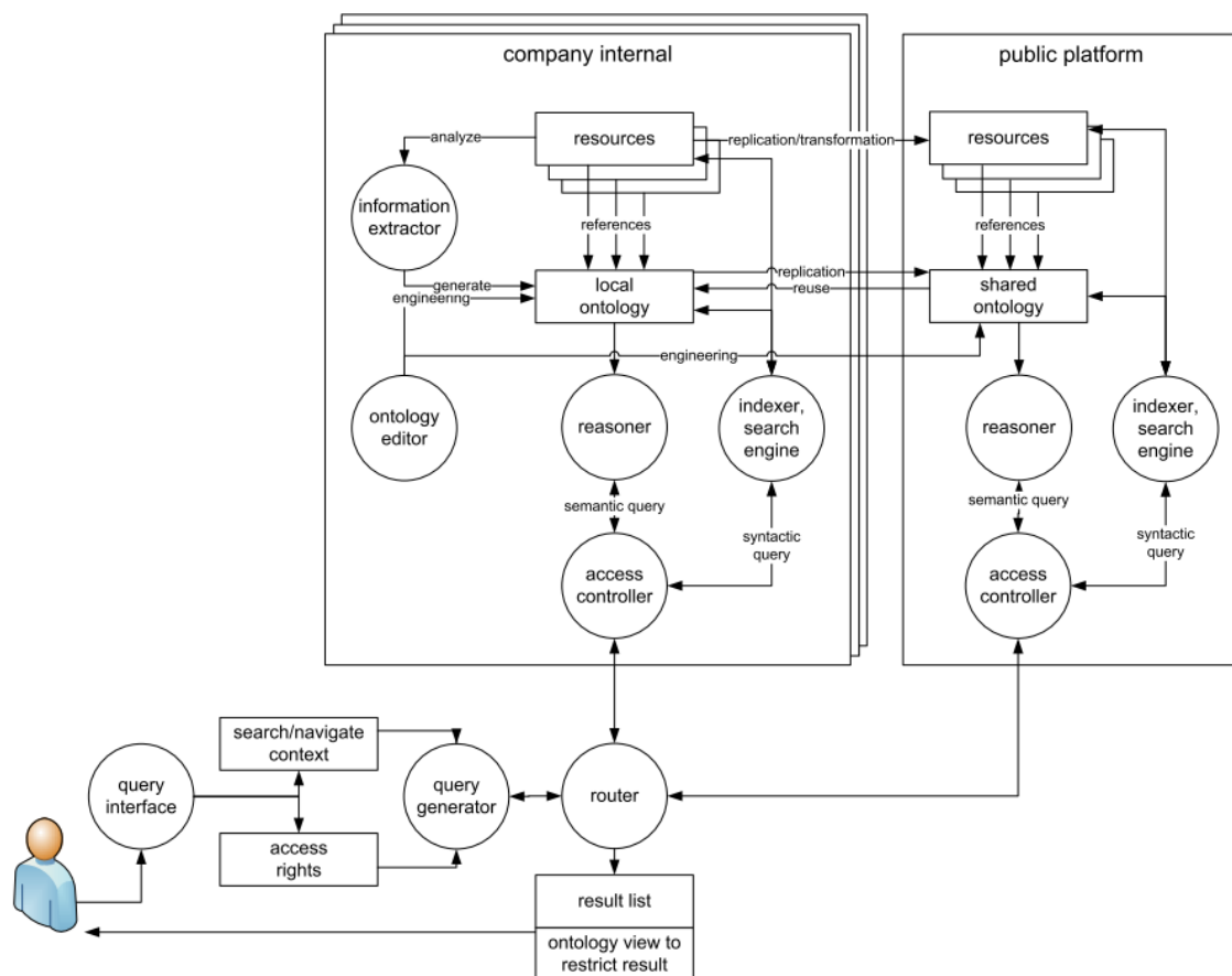
Abb. 4 : Gesamtarchitektur
