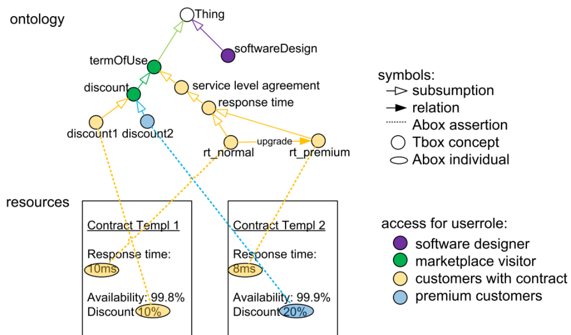
Abb. 1: Ressourcen, annotiert durch eine zugriffsbeschränkte Produktontologie
